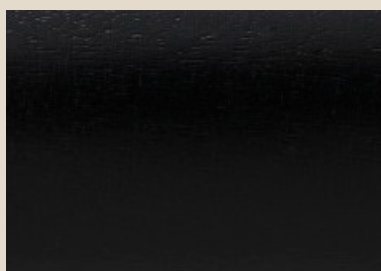
23 - Ébano
